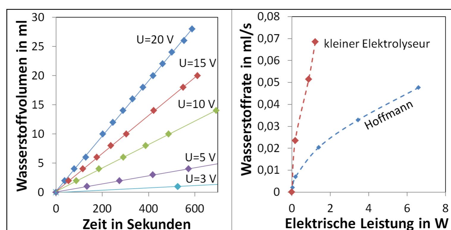
Abb 5: links: Produziertes Wasserstoffvolumen des Hoffmannschen Zersetzungsgenerators in ml nach einer gewissen Zeit für verschiedene Betriebsspannungen. Für 3V sind die Zeiten sehr lang, und wurden zur besseren Übersicht weggelassen. Die Steigung der Trendlinien gibt die Wasserstoffrate in ml/s. Rechts: die so gemessene, nicht lineare Wasserstoffrate abhängig von der elektrischen Eingangsleistung in W.
