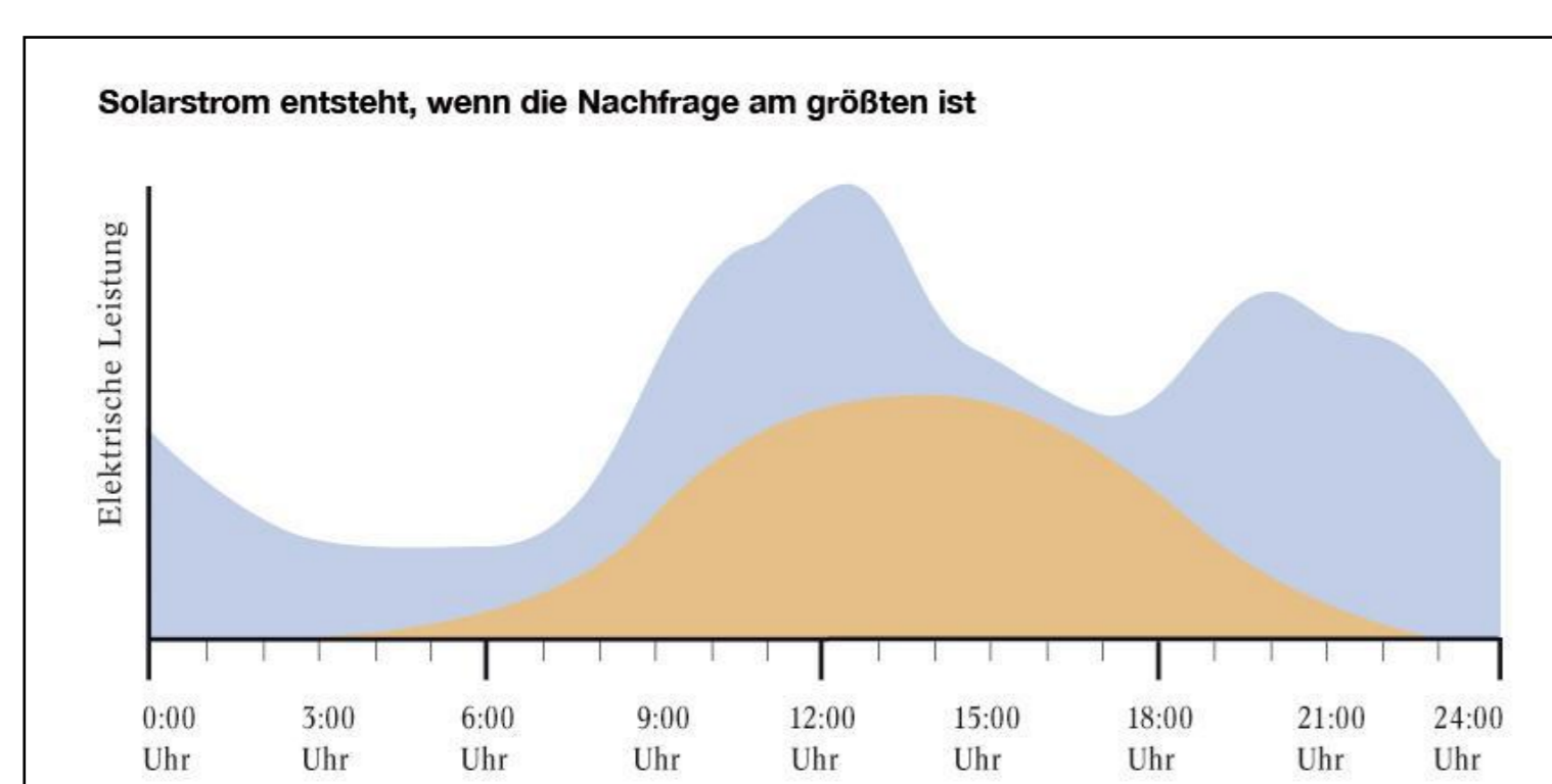
Abb 2: Blau: Stromverbrauch im Tagesverlauf, orange: Sonnenstromerzeugung an einem durchschnittlichen Sommertag in Deutschland [2]
